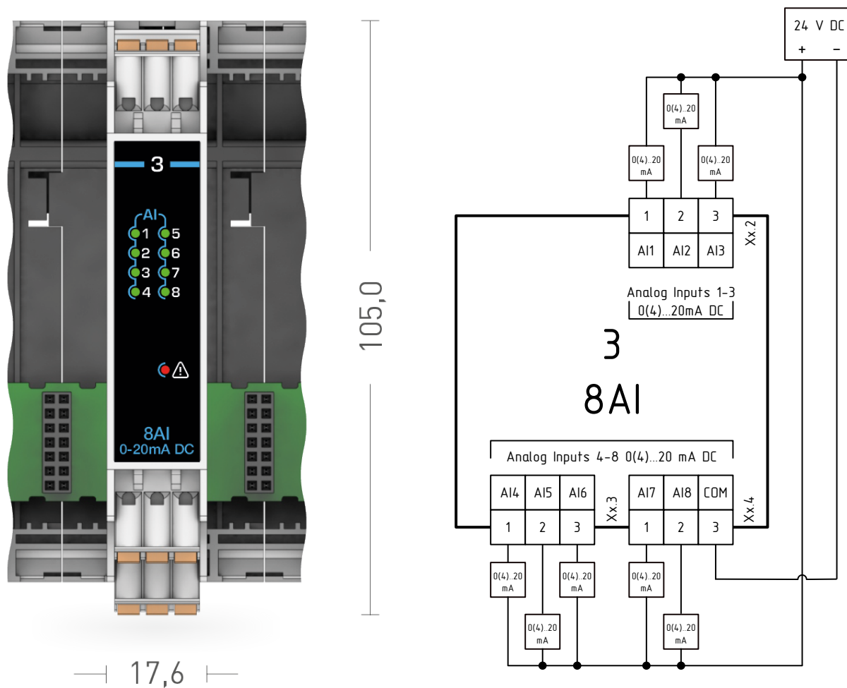
Рисунок 1.9 – Внешний вид и схема подключения модуля расширения MCU-3-8AI
