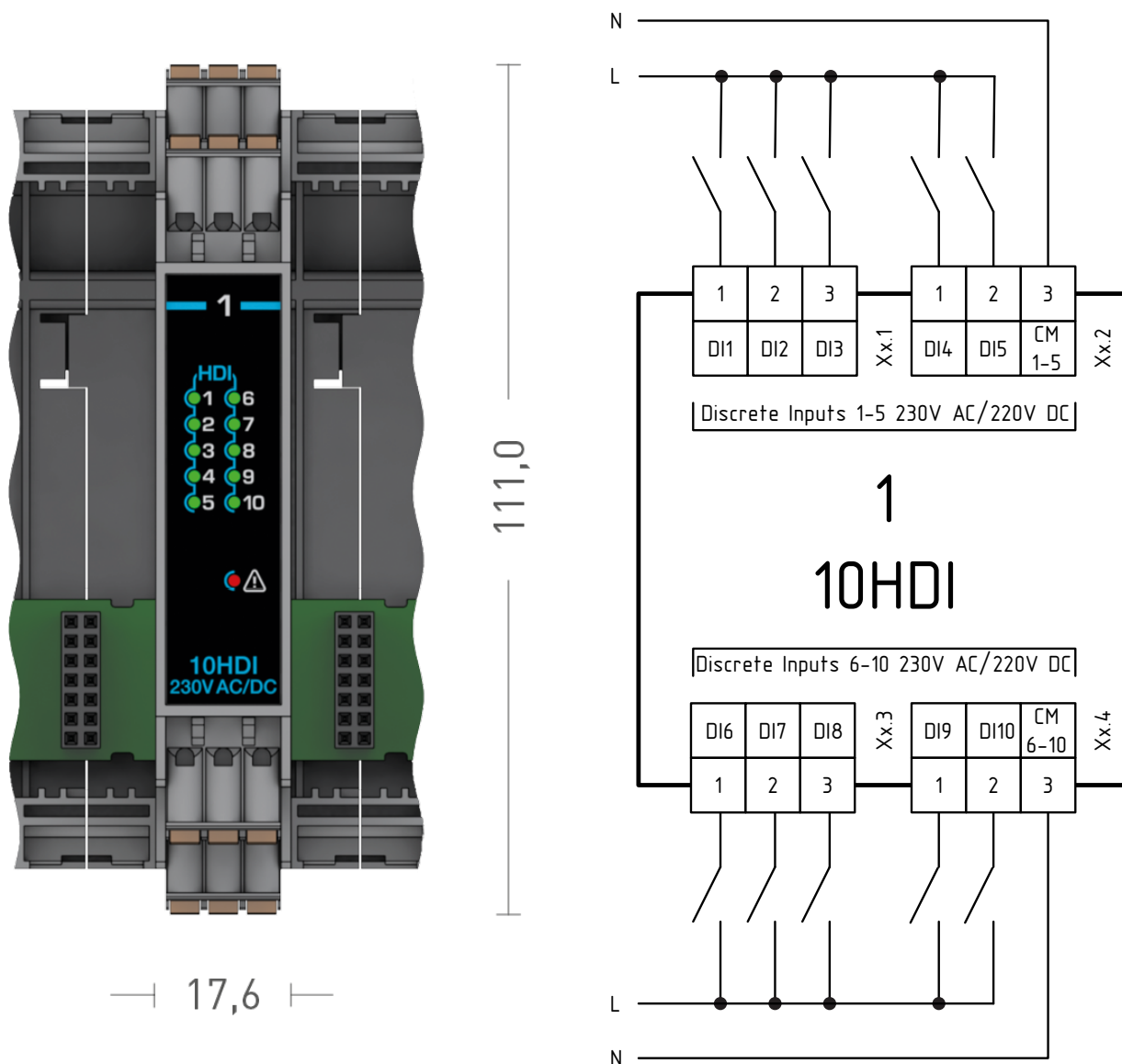
Рисунок 1.7 – Внешний вид и схема подключения модуля расширения MCU-1-10HDI
