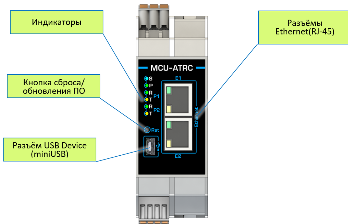
Рисунок 1.3 – Лицевая панель
