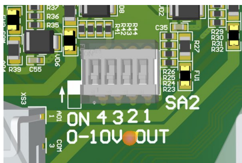
Рисунок 1.14 – Нумерация каналов и переключатели режимов на плате MCU-7-4AO
