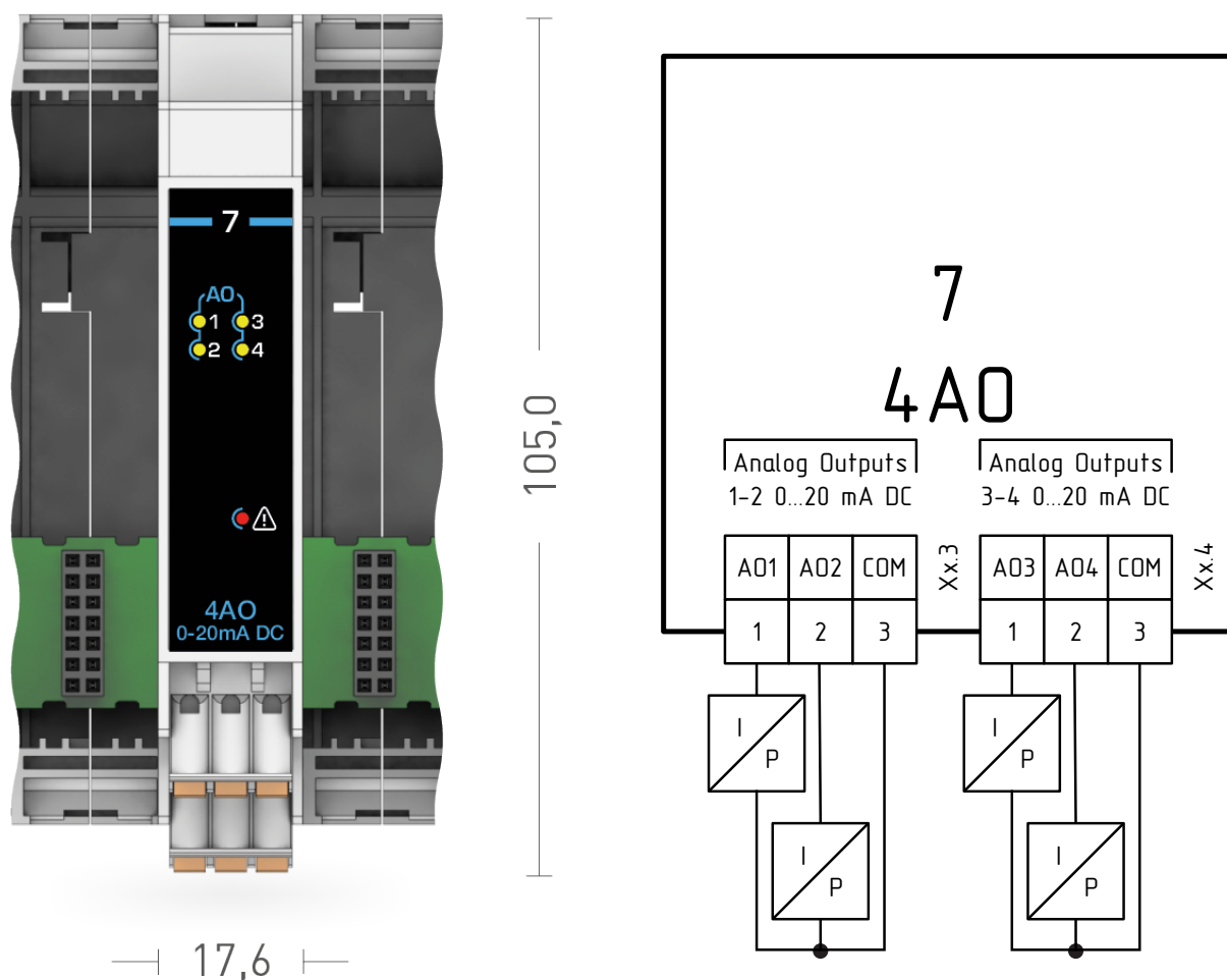
Рисунок 1.13 – Внешний вид и схема подключения модуля расширения MCU-7-4AO
