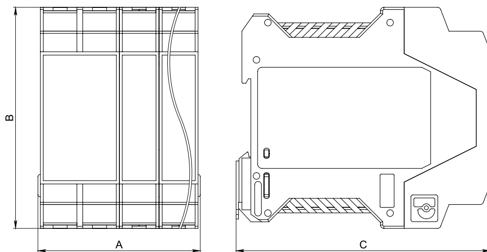
Рисунок 1.5 – Габаритные размеры устройства
