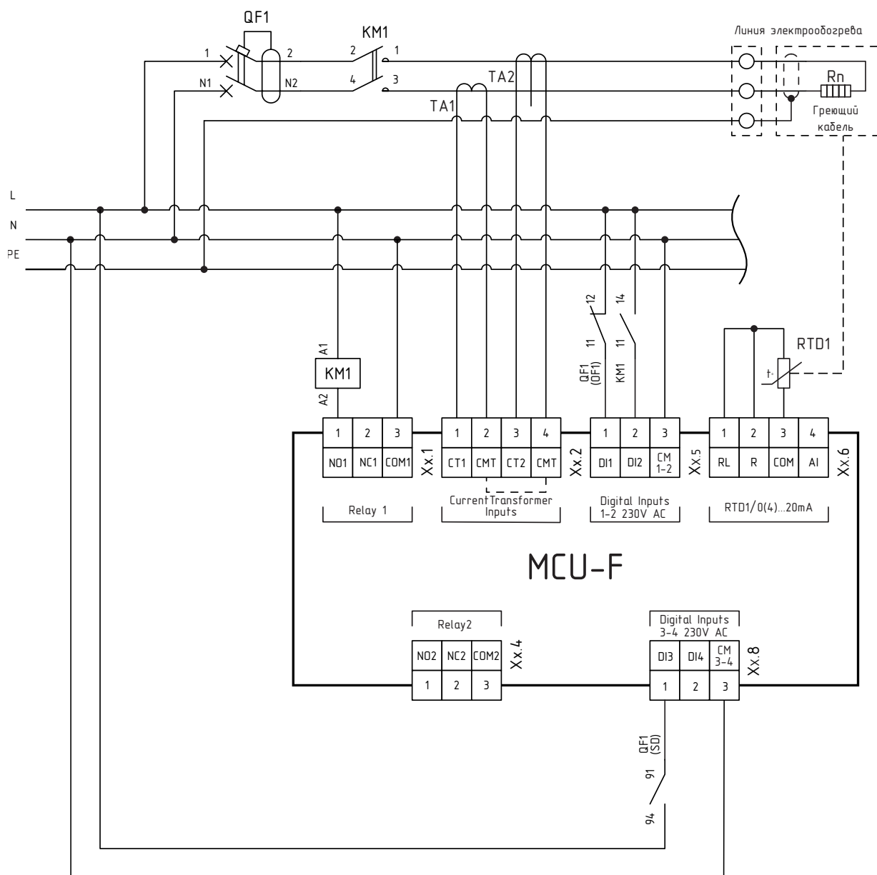
Рисунок 1.19 – Схема подключения модуля расширения MCU-F
