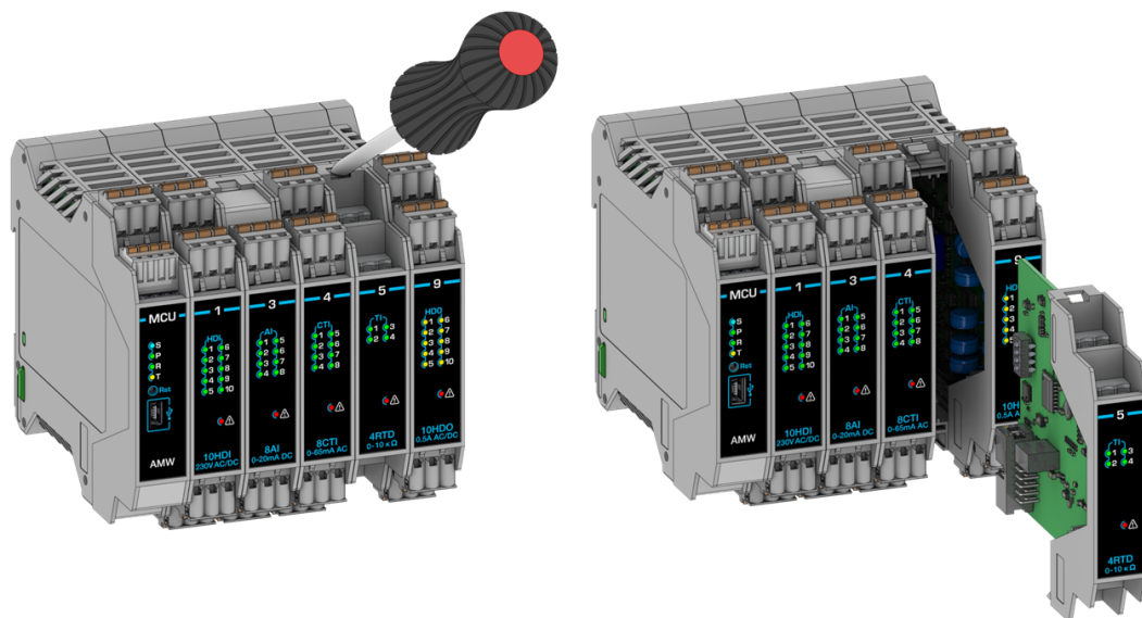
Рисунок 2.5 – Демонтаж модуля
