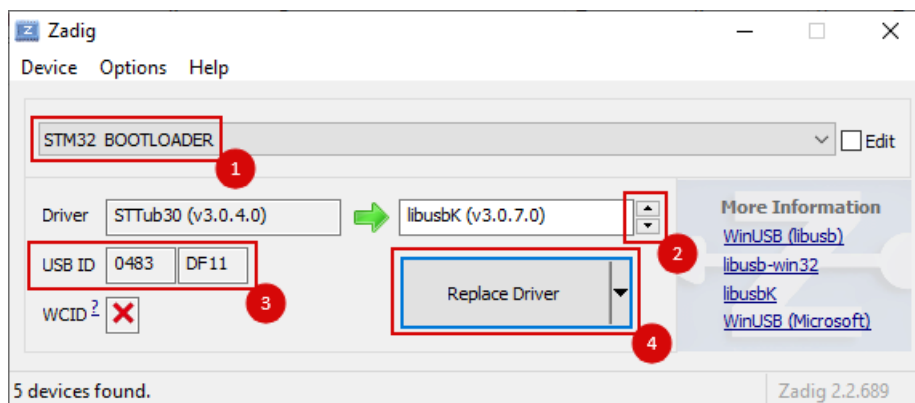
Рисунок Б.2 – Окно программы «Zadig»
