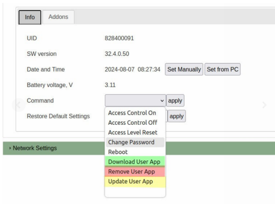
Рисунок Е.1 – Доступные действия с ППО
