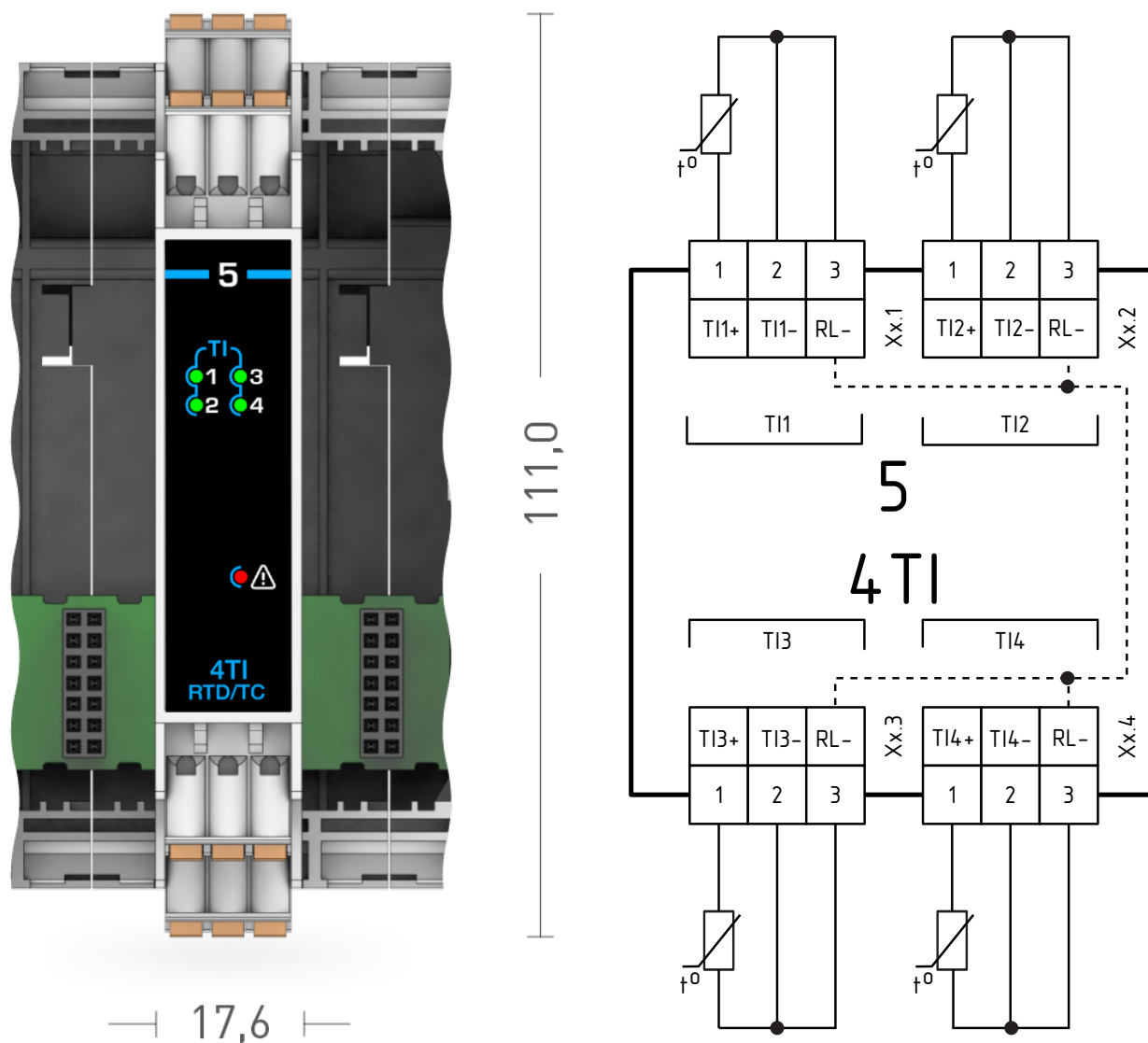
Рисунок 1.11 – Внешний вид и схема подключения модуля расширения MCU-5-4RTD
