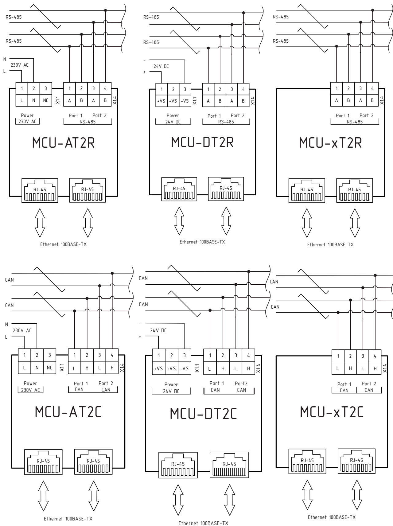
Рисунок 1.6 – Схемы подключения
