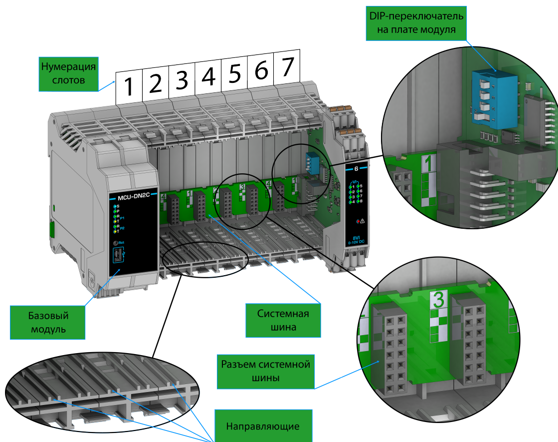
Рисунок 2.3 – Снятие разъемов с модуля
