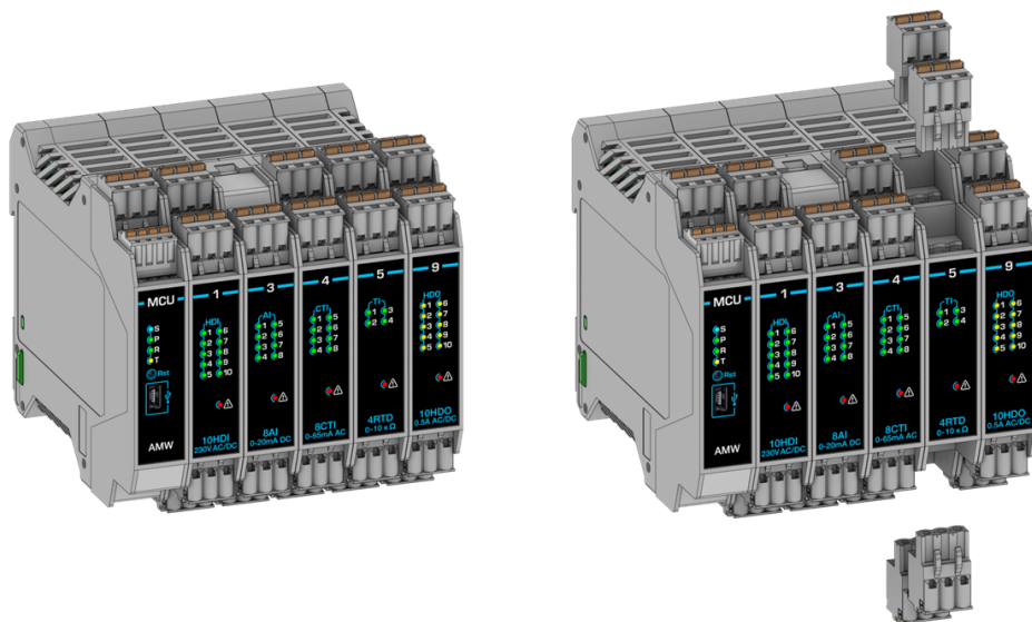
Рисунок 2.4 – Демонтаж модуля
