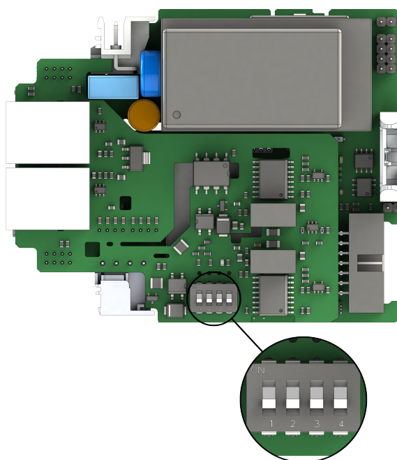
Рисунок 2.1 – Переключатели резисторов смещения
