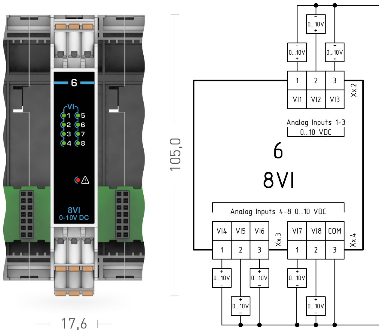
Рисунок 1.12 – Внешний вид и схема подключения модуля расширения MCU-6-8VI
