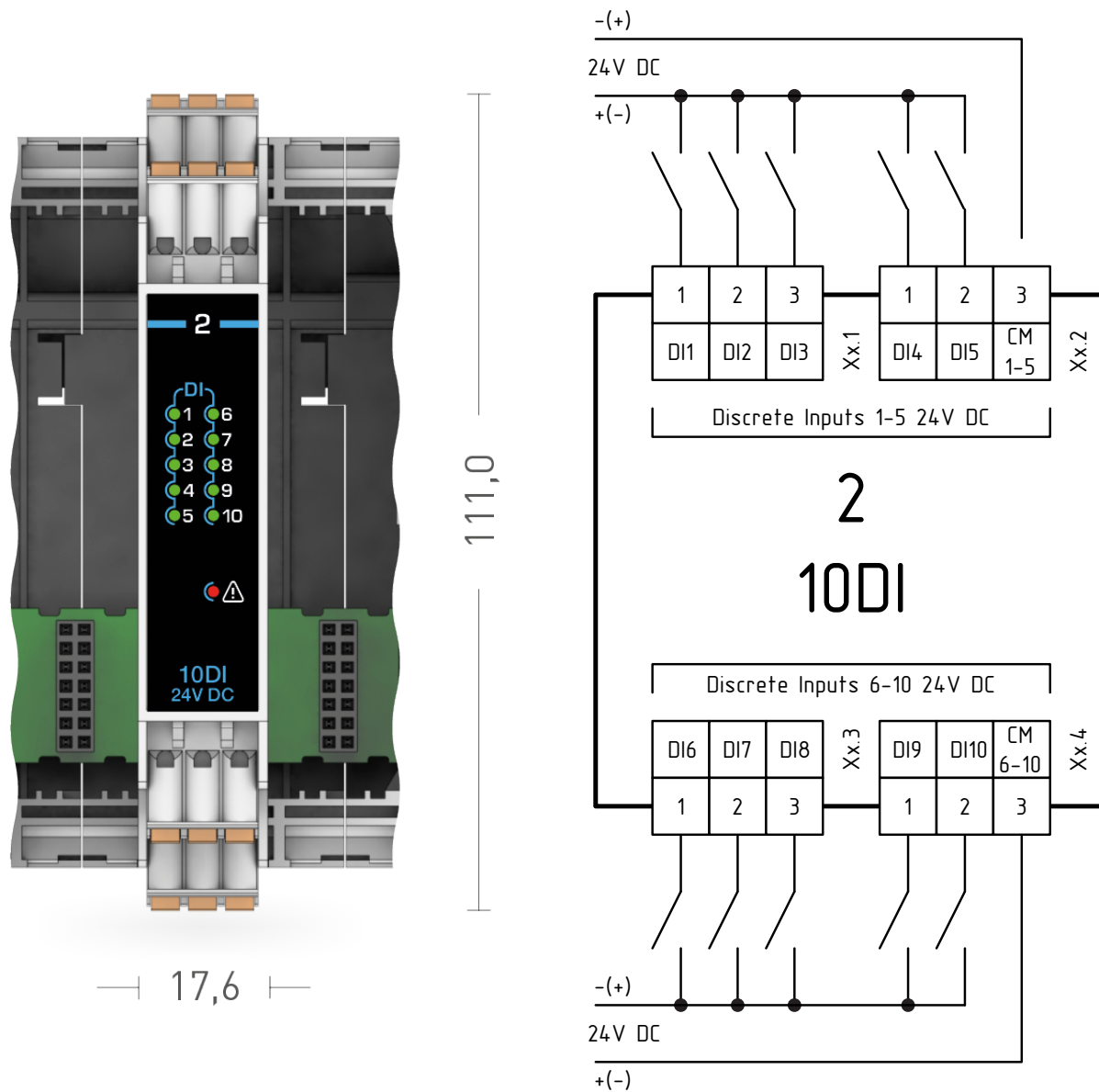
Рисунок 1.8 – Внешний вид и схема подключения модуля расширения MCU-2-10DI
