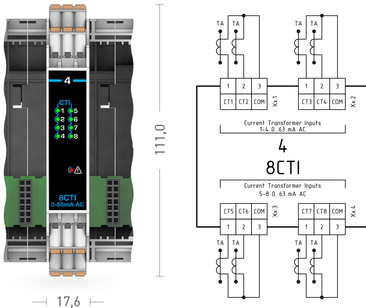
Рисунок 1.10 – Внешний вид и схема подключения модуля расширения MCU-4-8CTI
