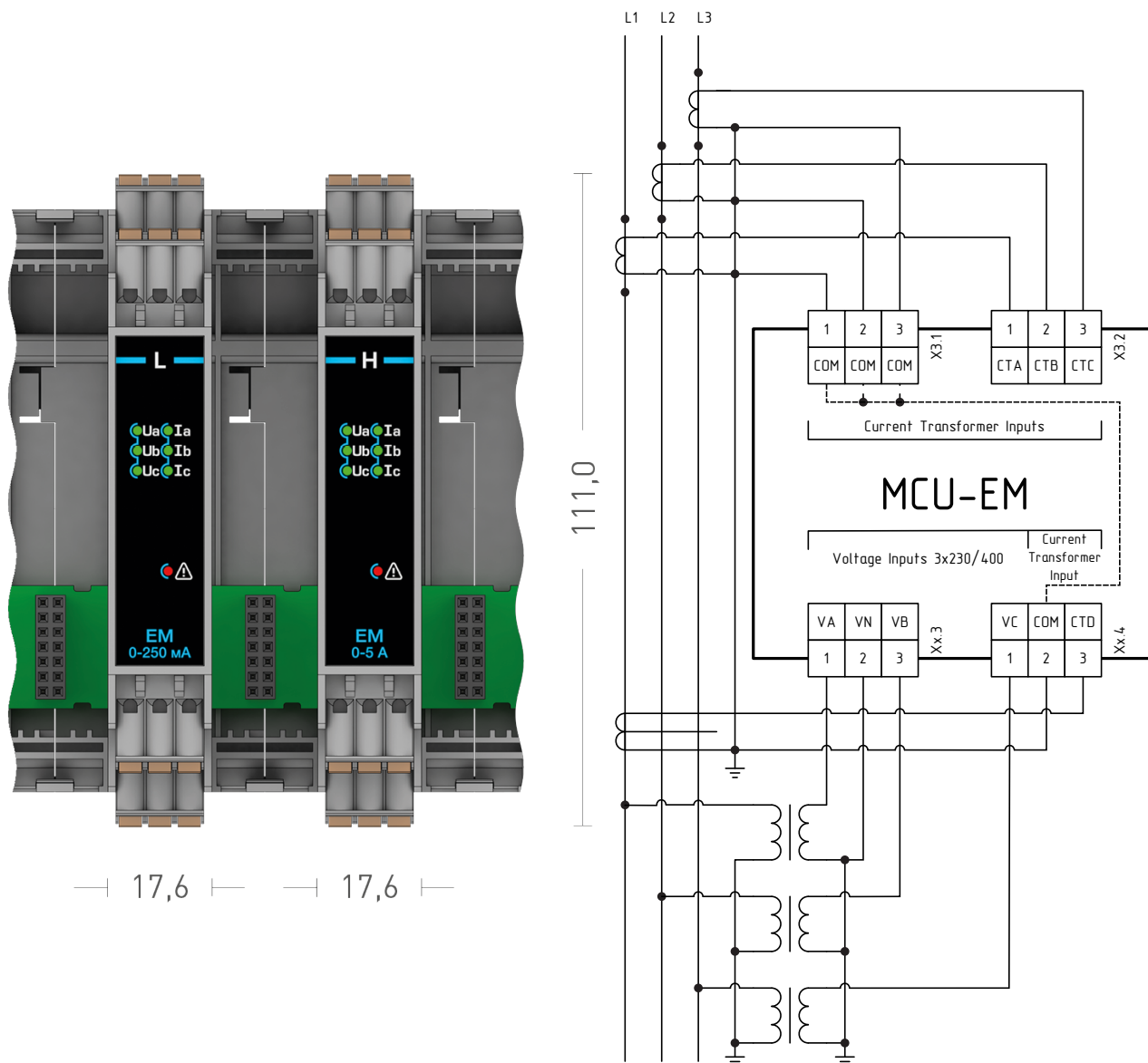
Рисунок 1.17 – Внешний вид и схема подключения модуля расширения EM
