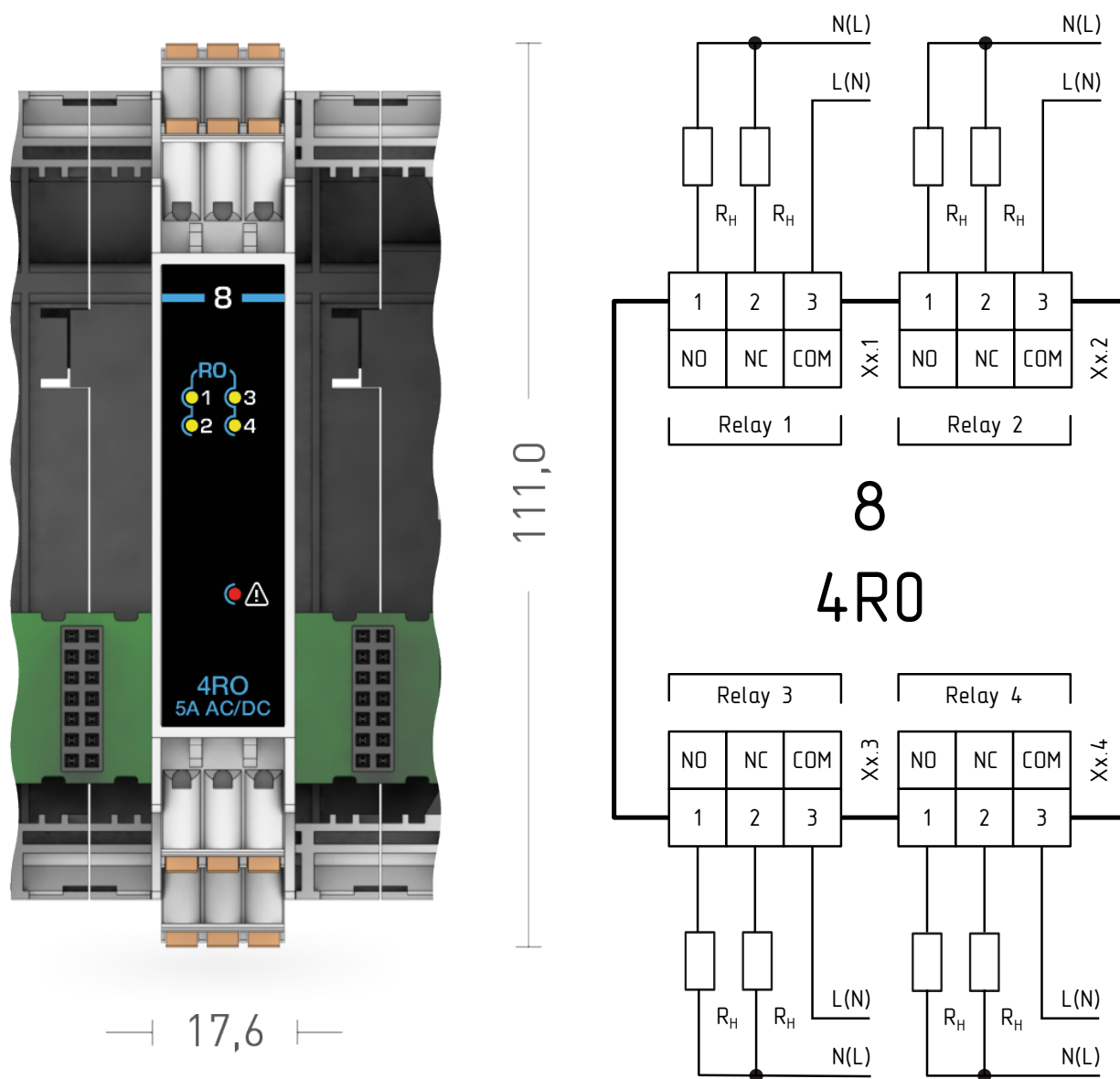
Рисунок 1.15 – Внешний вид и схема подключения модуля расширения MCU-8-4RO
