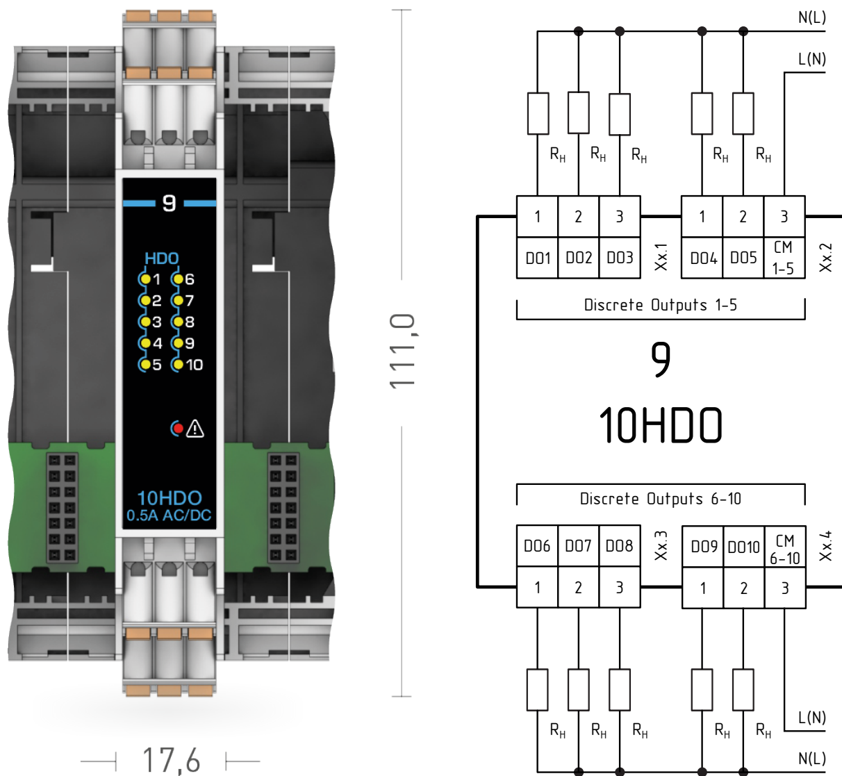
Рисунок 1.16 – Внешний вид и схема подключения модуля расширения MCU-9-10HDO
