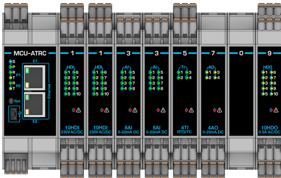
Рисунок 1.2 – Внешний вид устройства
