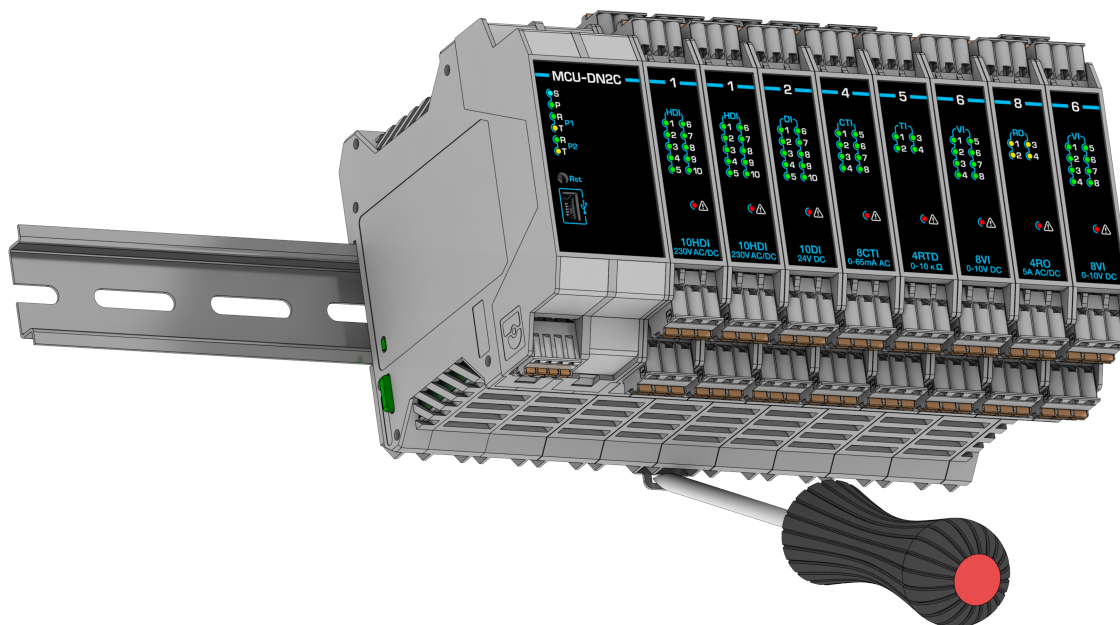
Рисунок 2.2 – Демонтаж устройства с DIN-рейки
