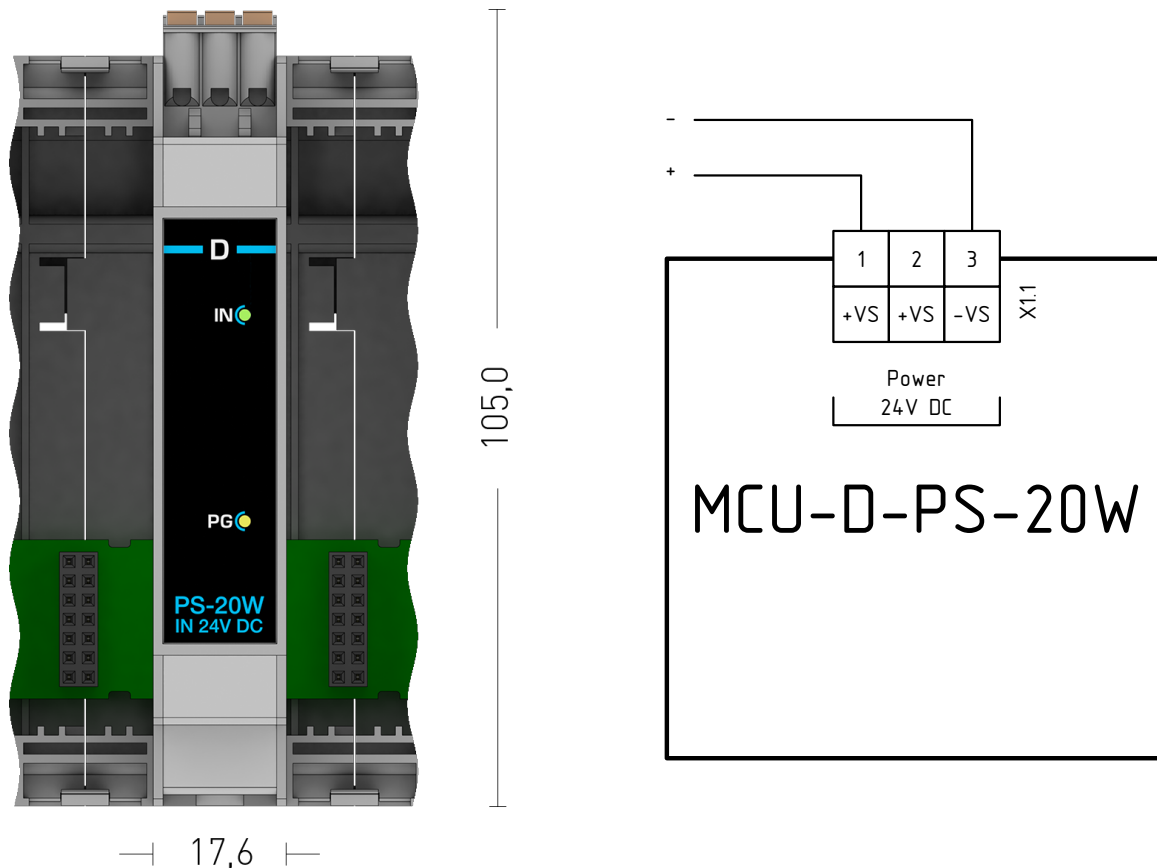
Рисунок 1.20 – Внешний вид и схема подключения модуля питания D-PS-20W
